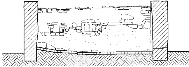
Εσωτερική Νότια Όψη
