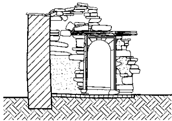
Εσωτερική Δυτική Όψη
